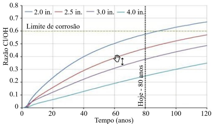
Figura 3. Evolução da relação cloreto/hidróxido ao longo do tempo e início esperado de corrosão do aço em diferentes profundidades com reparos mínimos para preservar o concreto como está.
