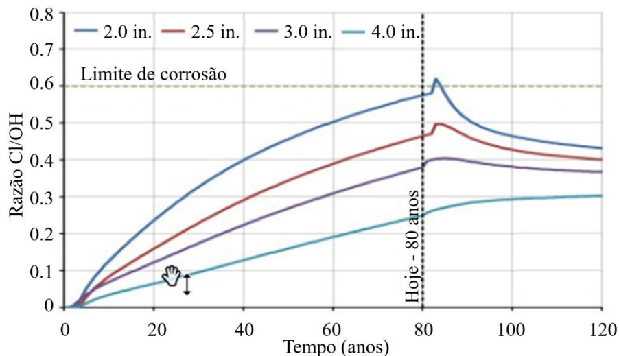
Figura 4. Evolução da relação cloreto/hidróxido ao longo do tempo e início esperado de corrosão da armadura em diferentes profundidades usando estratégia de reparo robusta.
