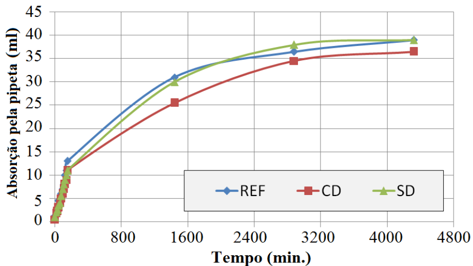
Figura 8. Absorção pelo método da pipeta para a série de referência e as duas formas de adição de NTC.
