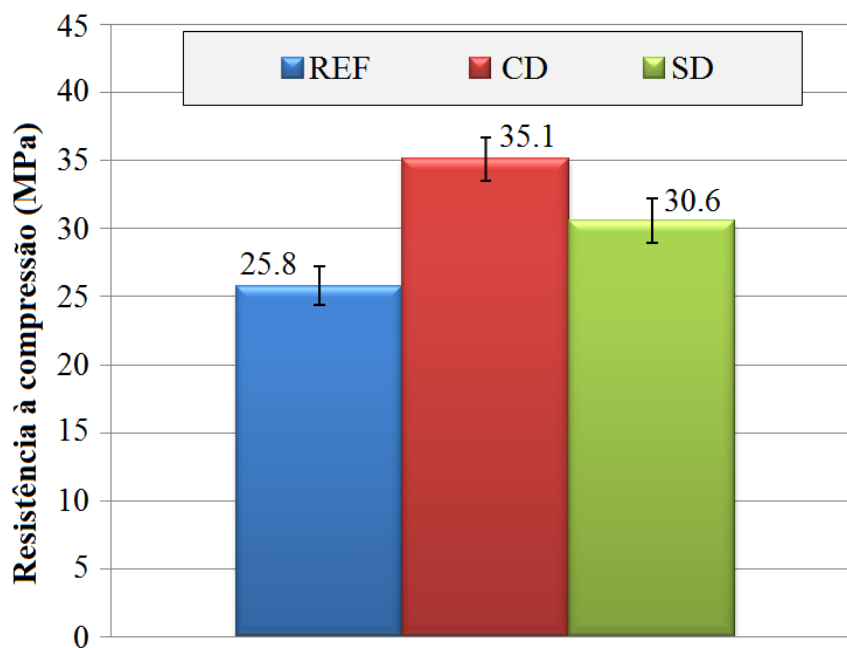
Figura 5. Resistência à compressão (MPa) para a série de referência e as duas formas de adição de NTC.
