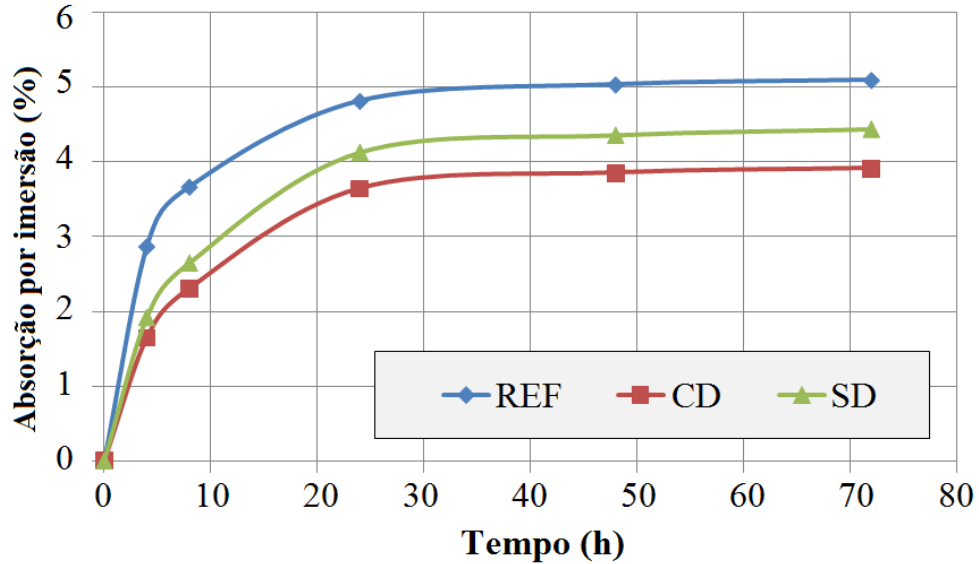
Figura 7. Absorção por imersão (%) X tempo (h) para a série de referência e as duas formas de adição de NTC.
