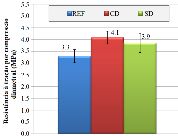
Figura 6. Resistência à tração por compressão diametral para a série de referência e as duas formas de adição de NTC.
