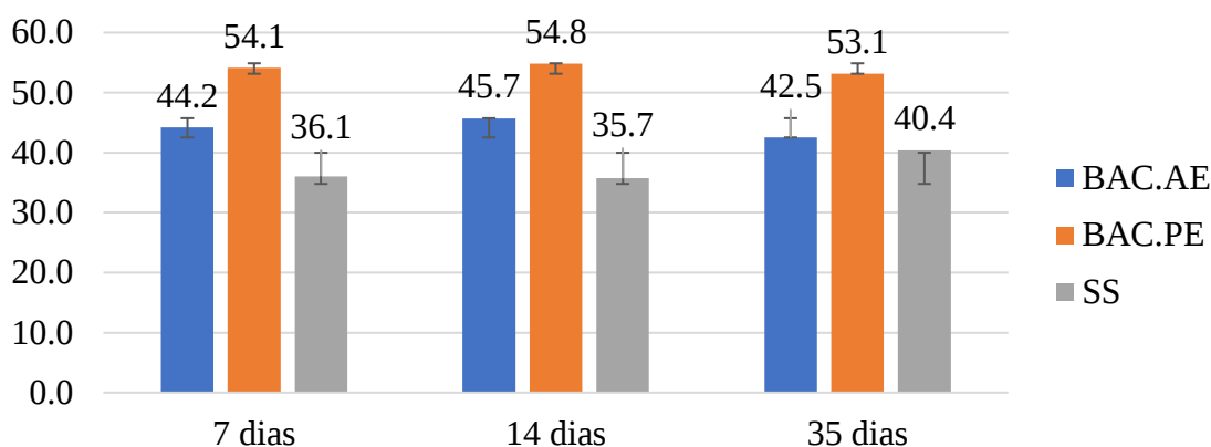
Figura 4. Resistência à compressão média das amostras.
