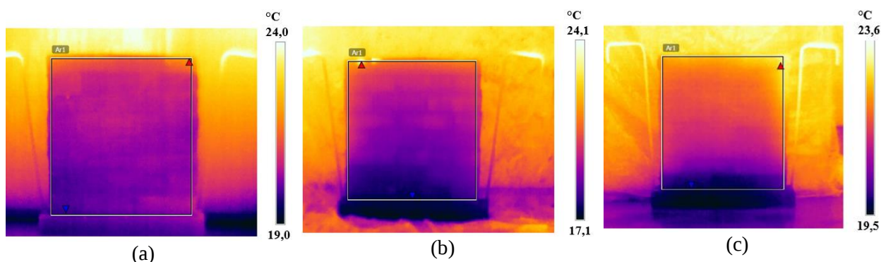
Figura 12. Amostra PB2: a) parede seca; b) parede úmida; c) parede aos 28 dias
