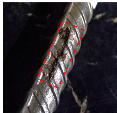
Figura 21. Perda de massa das barras de aço (L1).
