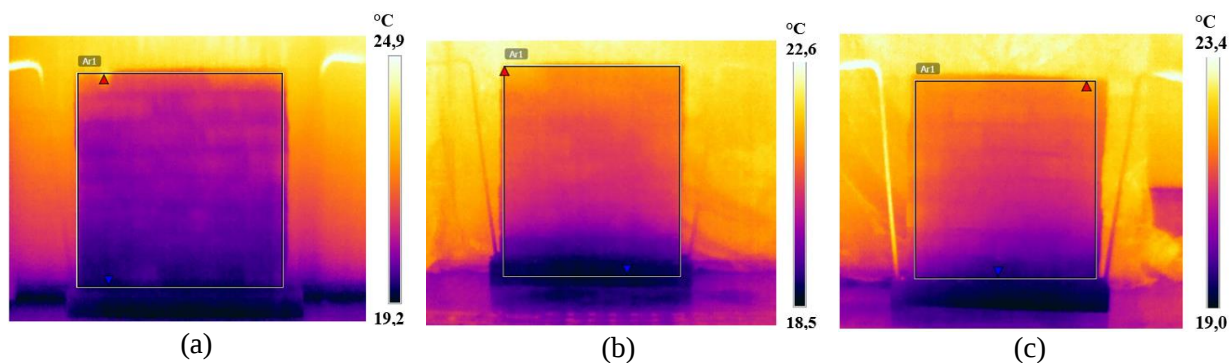
Figura 9. Amostra PA1: a) parede seca; b) parede úmida; c) parede aos 28 dias
