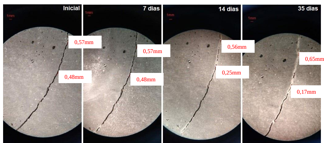
Figura 6. Autocicatrização no traço BAC.AE – Amostra 2.
