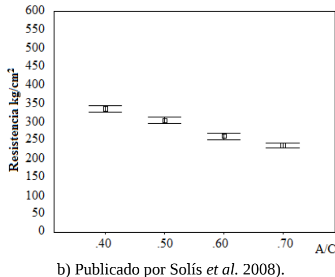
Figura 2. Comparación de los promedios de las resistencias a 28 días medidas en este estudio con los reportados en estudio previo con los mismos materiales (95% de confianza).
