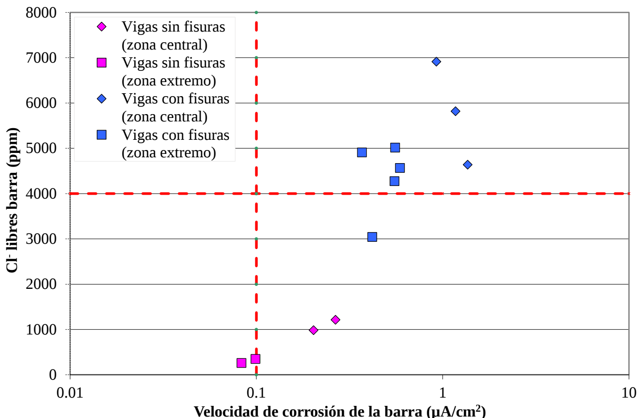
Figura 10. Concentración de ión cloruro a nivel de la armadura vs. velocidad de corrosión, vigas de concreto con y sin fisuras (Hernández, 2009)
