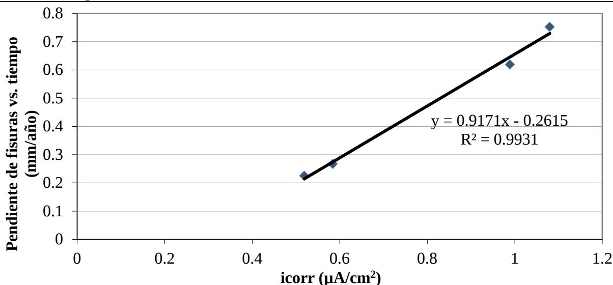
Figura 8. Pendiente promedio de anchos de fisuras en el tiempo vs. velocidad de corrosión del refuerzo (Hernández, 2009)
