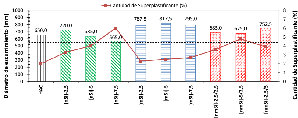
Figura 2. Diámetro de escurrimiento ( d_f ) (mm) y cantidad de superplastificante.
