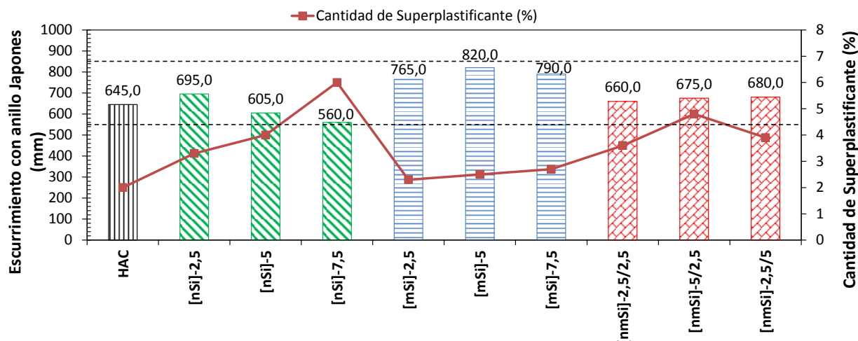
Figura 5. Diámetro de escurrimiento con anillo japonés (cm) y cantidad de superplastificante.
