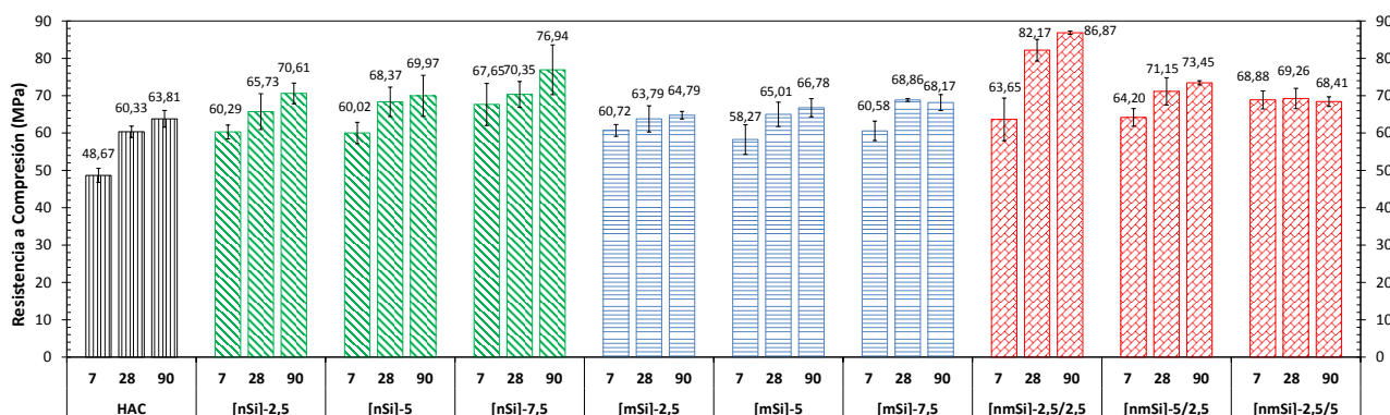
Figura 6. Resistencia a Compresión (MPa)
